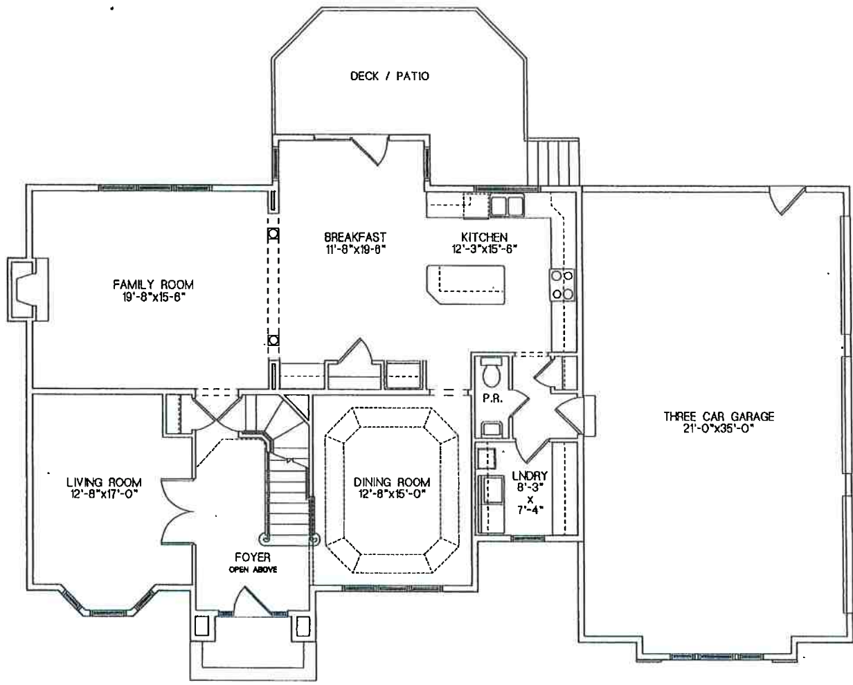
FIRST FLOOR PLAN 66'-0" (W) x 43'-0" (D) 1472.21 SQ. FT.
